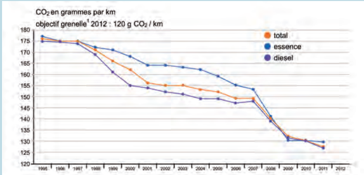
Document 1 - Émission spécifique de CO 2 des voitures vendues
